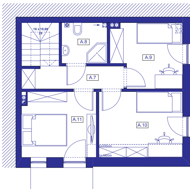
RZUT PIĘTRA
