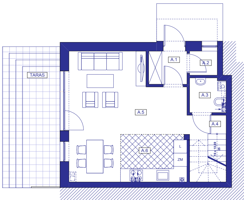
RZUT PARTERU
