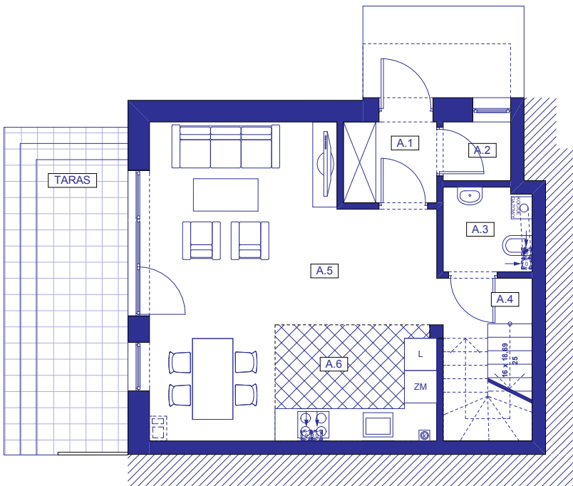
RZUT PARTERU
